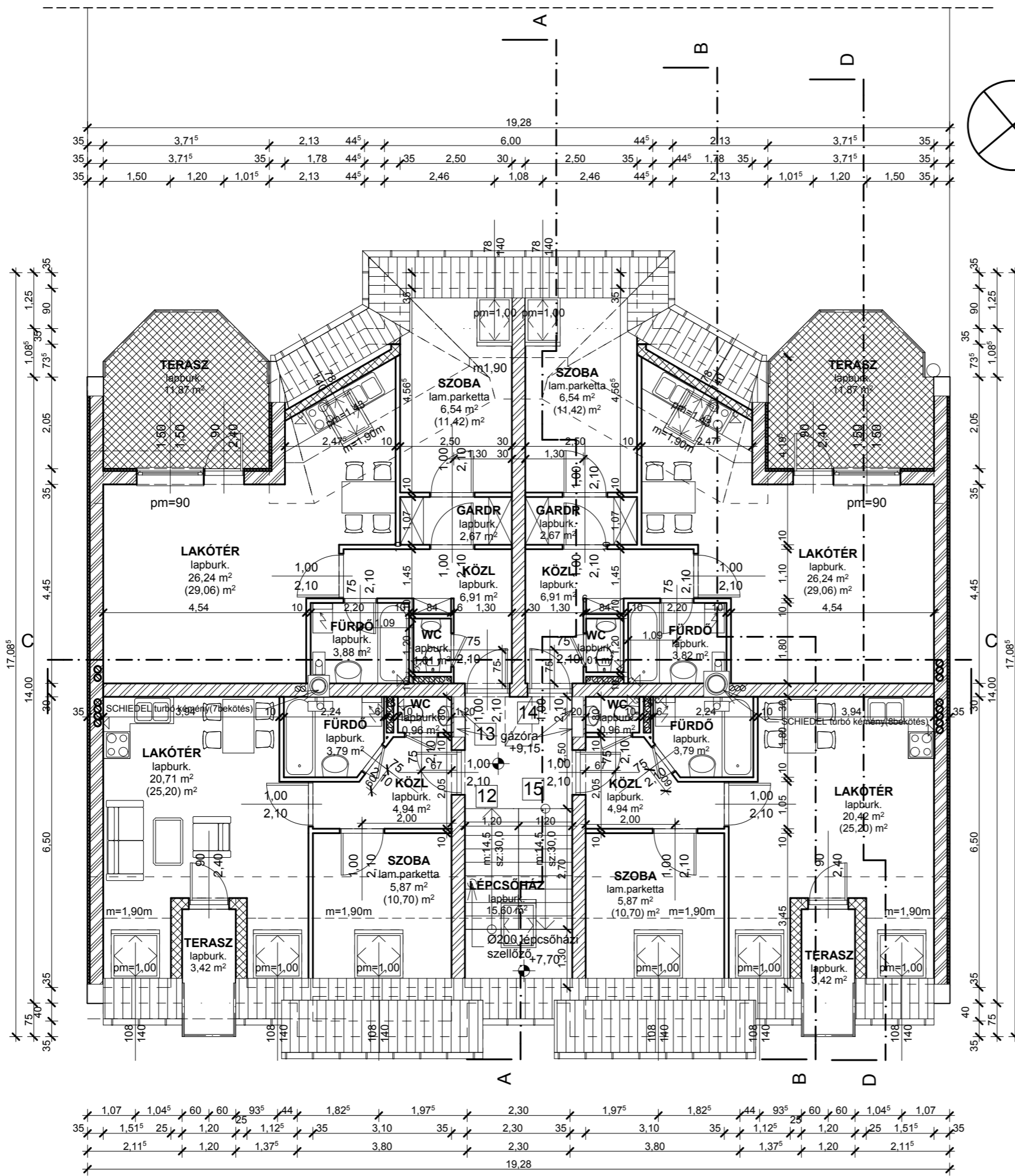
TETŐTÉRI ALAPRAJZ M 1:100
