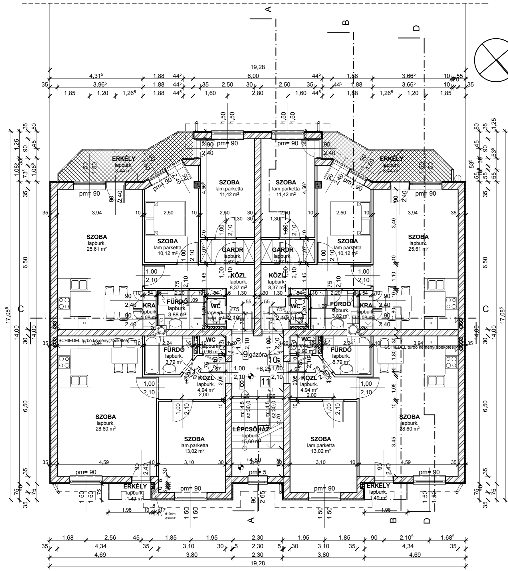
II. EMELETI ALAPRAJZ M 1:100
