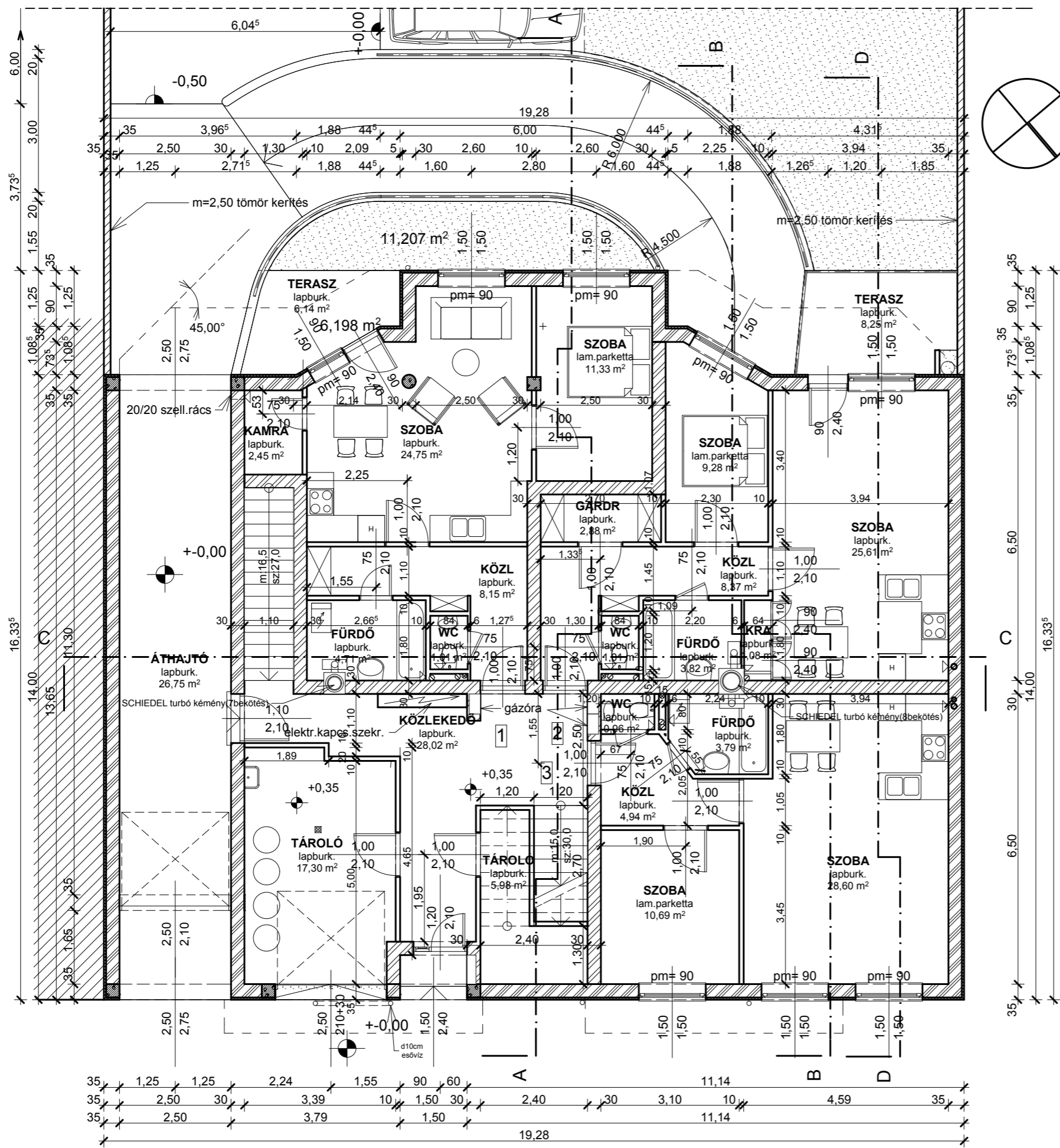
FÖLDSZINTI ALAPRAJZ M 1:100
